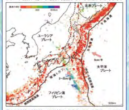
震央(1998年~2007年、M4以上)は、気象庁による。矢印は、ユーラシアプレートに対する太平洋プレートとフィリピン海プレートの相対的な進行方向と速さを示す。太い実線はプレート境界、破線は不明瞭なプレート境界を示す。文部科学省「地震がわかる! Q&A」
